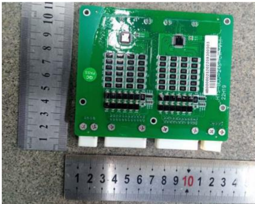
Photo 3 电池组保护板正面 Front view of PCM
