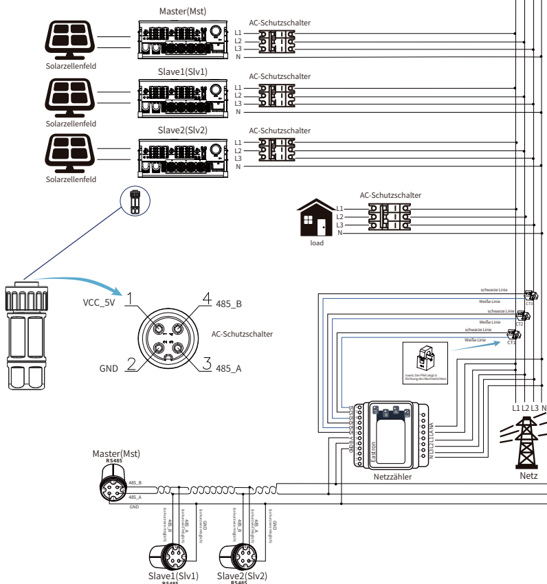
Abb. 7.25 Anschlussplan (Dreiphasenstrom)
