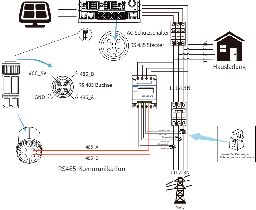
Abb. 7.14 Anschlussplan des CHINT-Zählers
