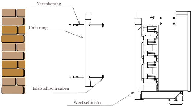
Abb. 4.5 Installation des Wechselrichters
