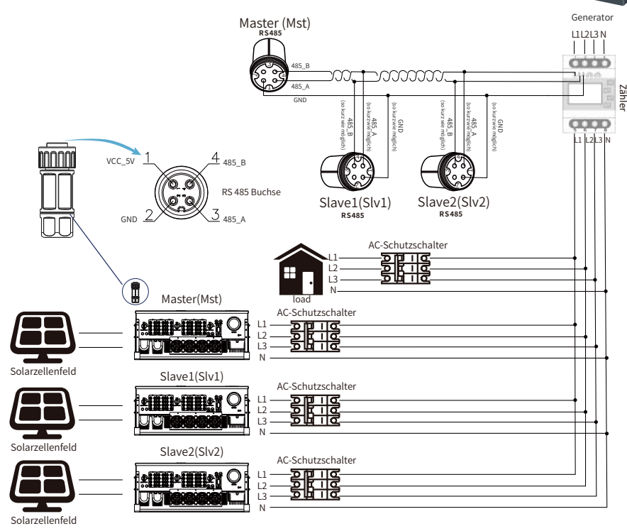
Abb. 7.23 EASTRON Anschlussplan (Die Durchleitungstabelle)
