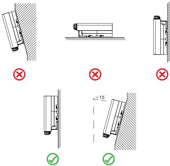
Abb. 4.2 Einbauwinkel
