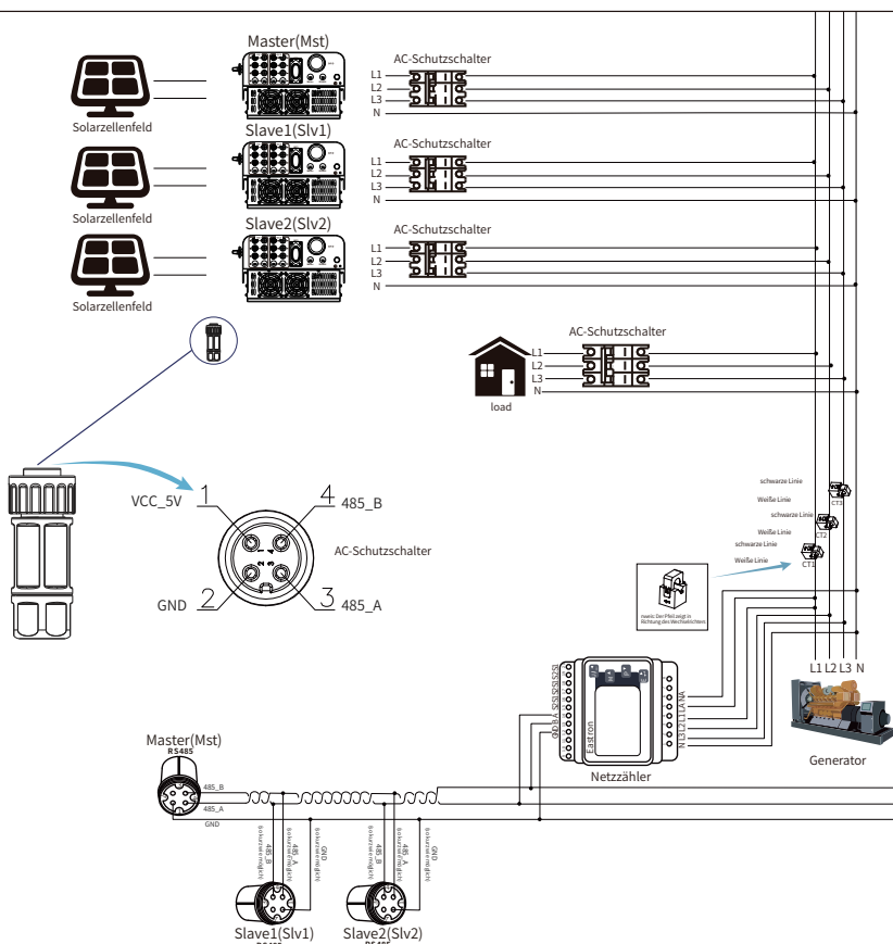
Abb. 7.25 Anschlussplan (Dreiphasenstrom)
