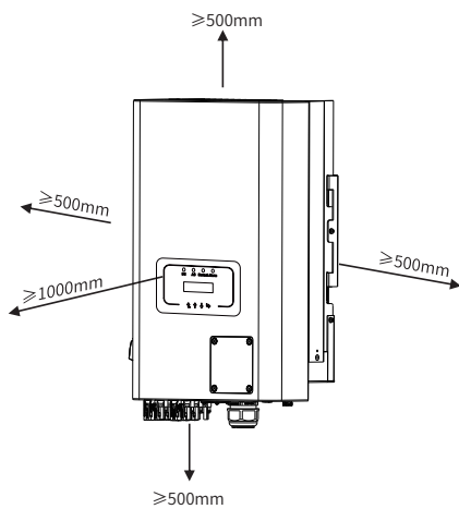
Abb. 4.3 Einbaulücke
